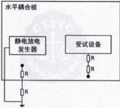
图6 被测设备连接图
