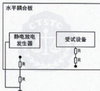
图 6 被测设备连接图
