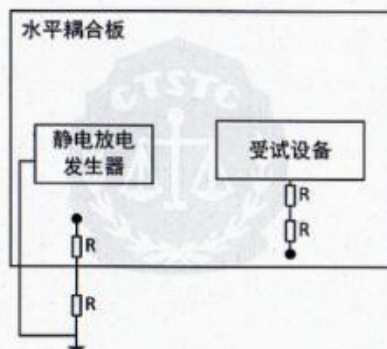
图6 被测设备连接图
