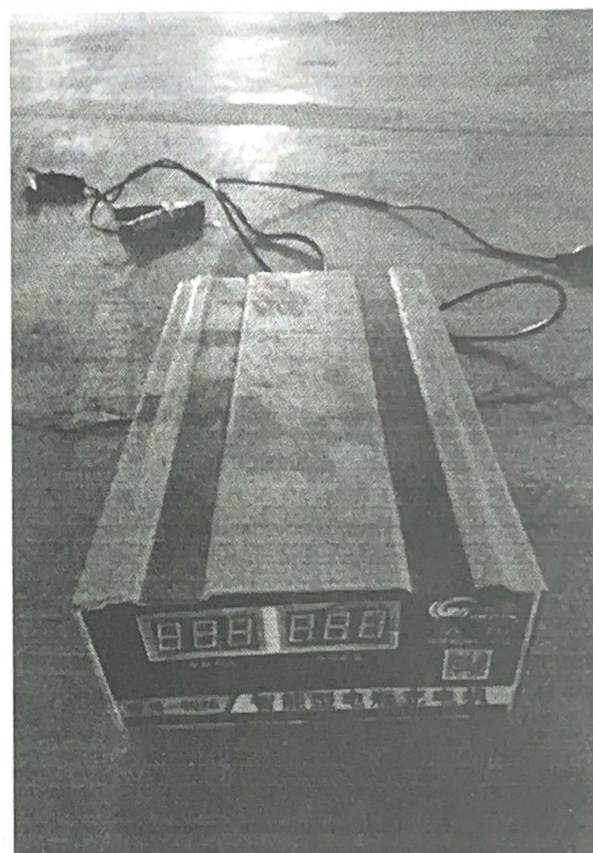
电瓶充电机
